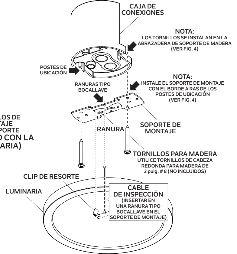
Fig. 3 INSTALACIÓN EN CAJA DE CONEXIONES DE VENTILADOR DE TECHO EN FORMA DE L
